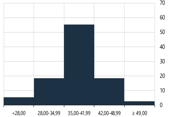
Grafik 3: 12 Ay Sonrası TÜFE Nokta Tahminlerinin Dağılımı (%)
